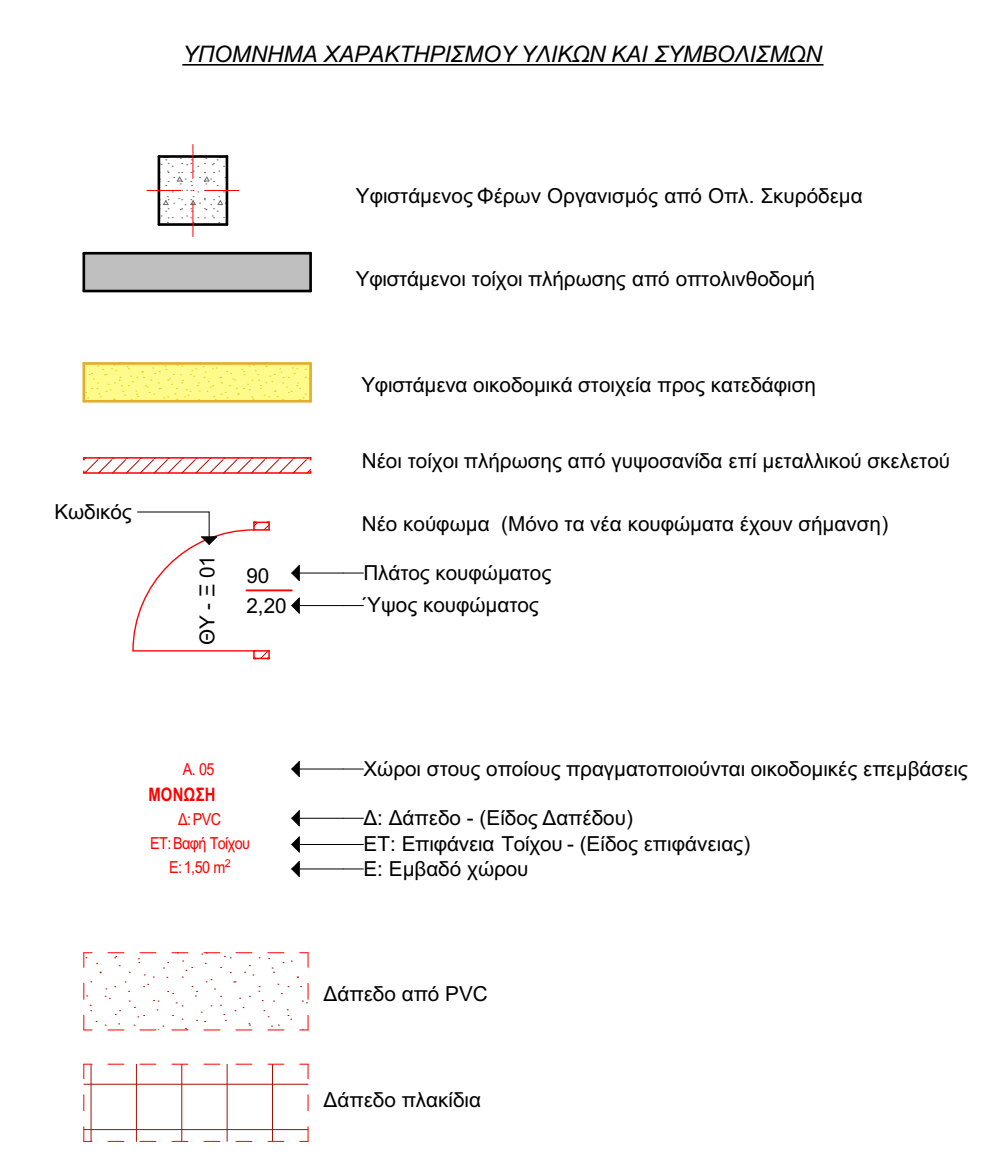
ΦΕ-04 Κλειδα 1:200
