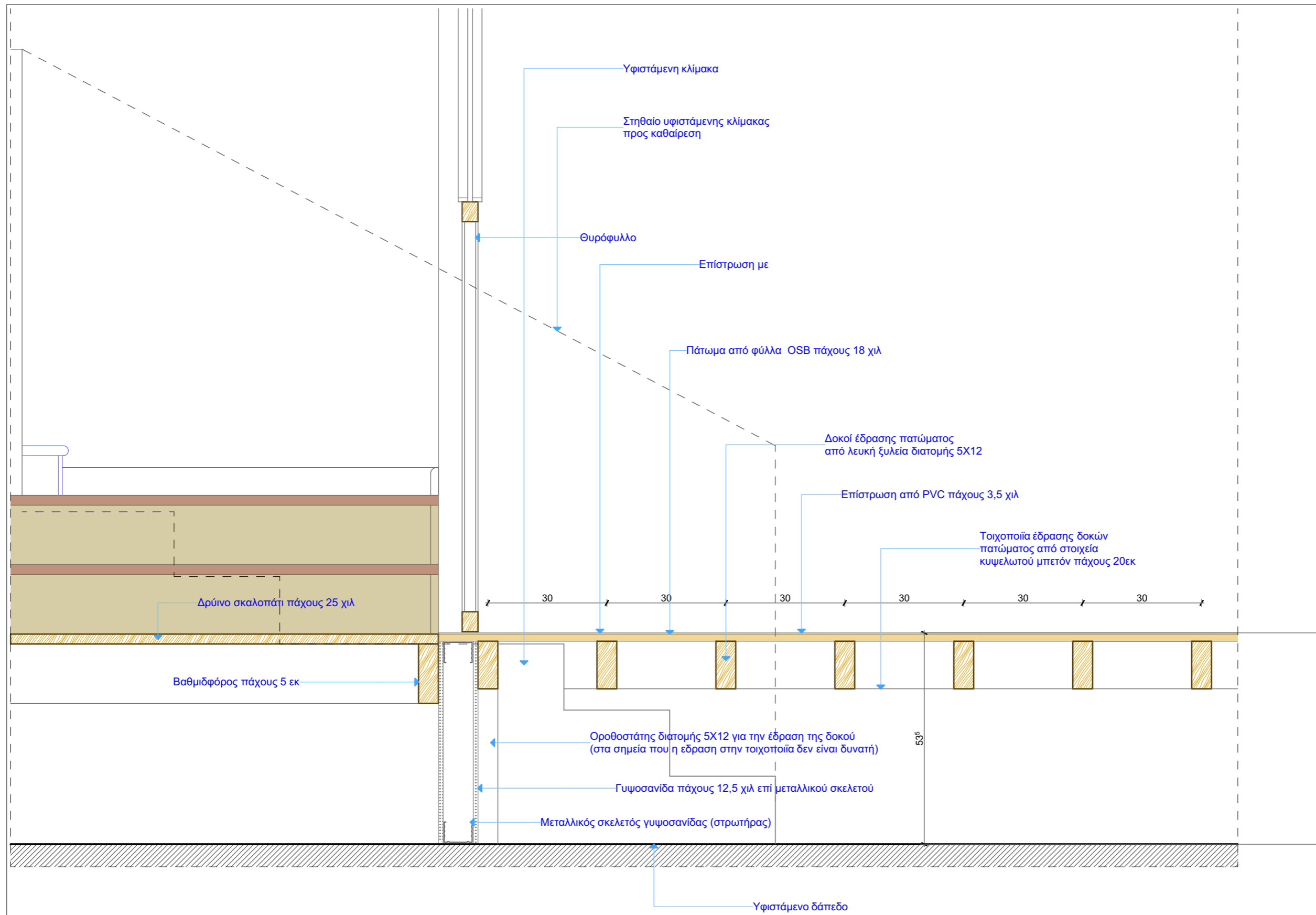
Λεπτομέρεια συναρμογής πατώματος με ξύλινη κλίμακα
