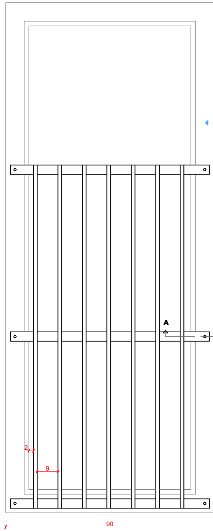
ΦΕ-10 Λεπτομέρεια κιγκλιδώματος σε εξωστόθουρα αλουμινίου 1:10
