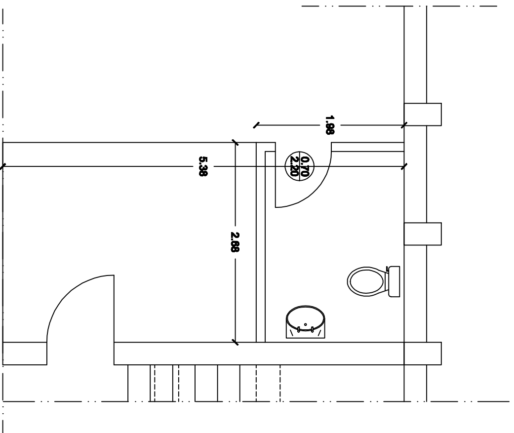
Υπόγειο Υπάρχουσα κατάσταση
