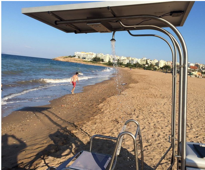
Εικόνα 13 Προσαρμοσμένη ντουζιέρα σε διάταξη για την αυτόνομη πρόσβαση ΑμεΑ στη θάλασσα
