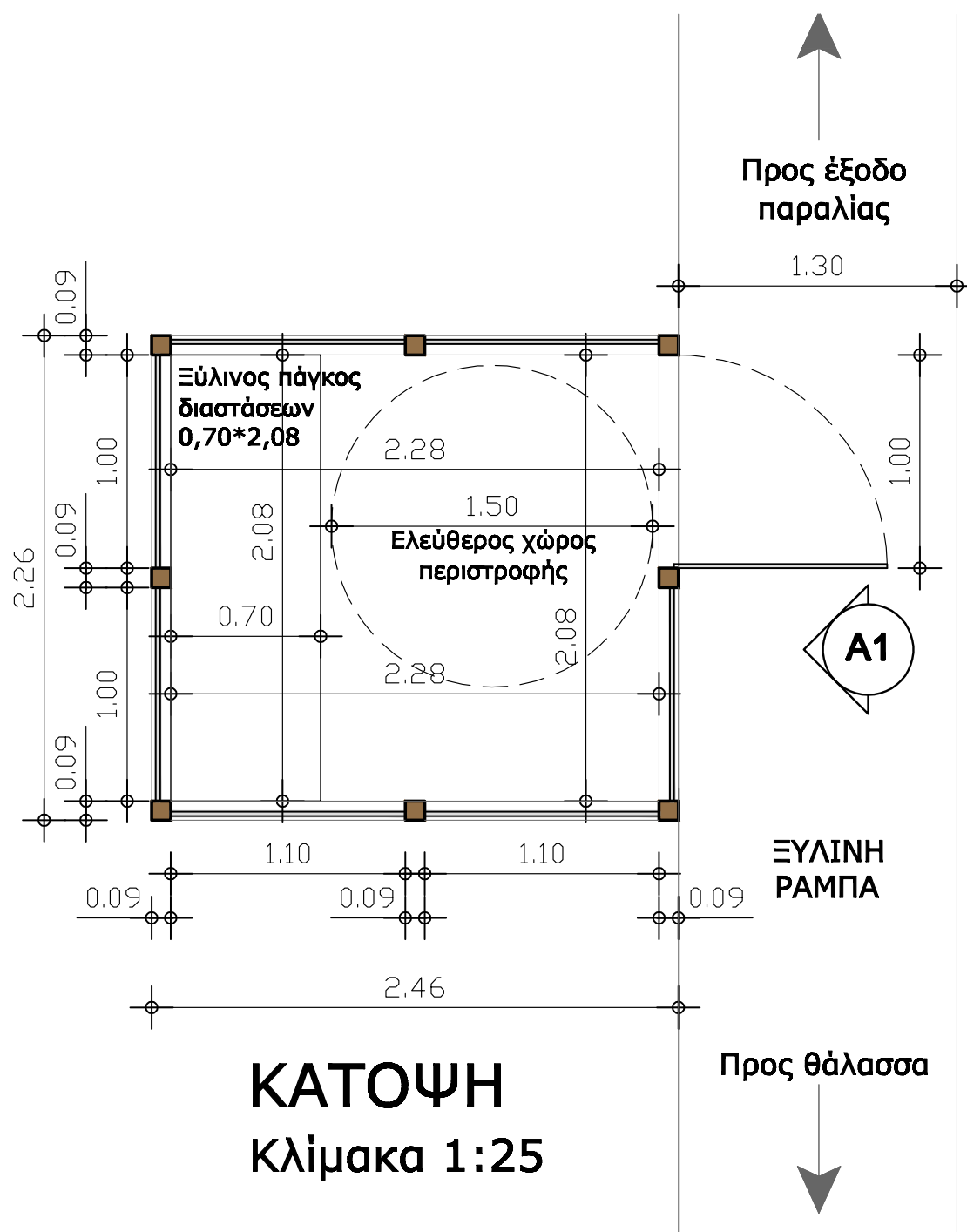
Εικόνα 10 Κάτοψη μη μόνιμο συναρμολογούμενο αποδυτήριο για ΑμεΑ
