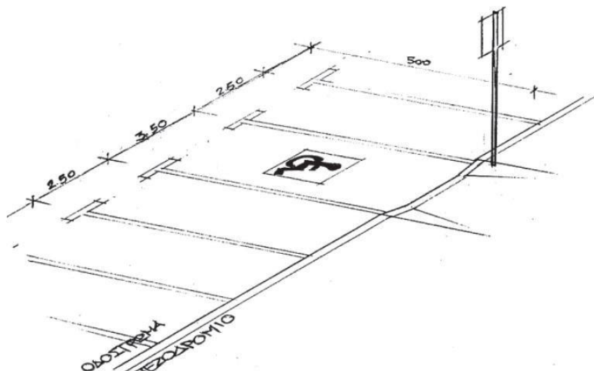
Εικόνα 6 Ειδικά διαμορφωμένη θέση στάθμευσης για ΑμεΑ (ΕΛΟΤ 1439 2013).
