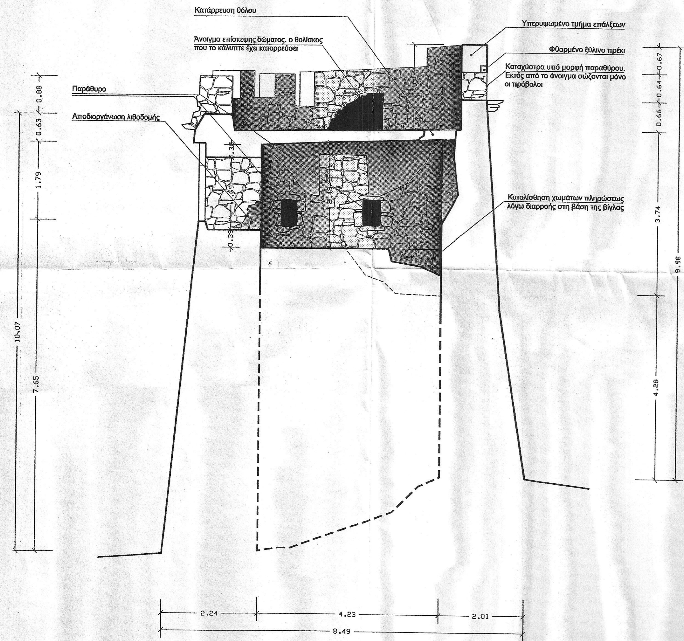
ΤΟΜΗ 1 - 1
