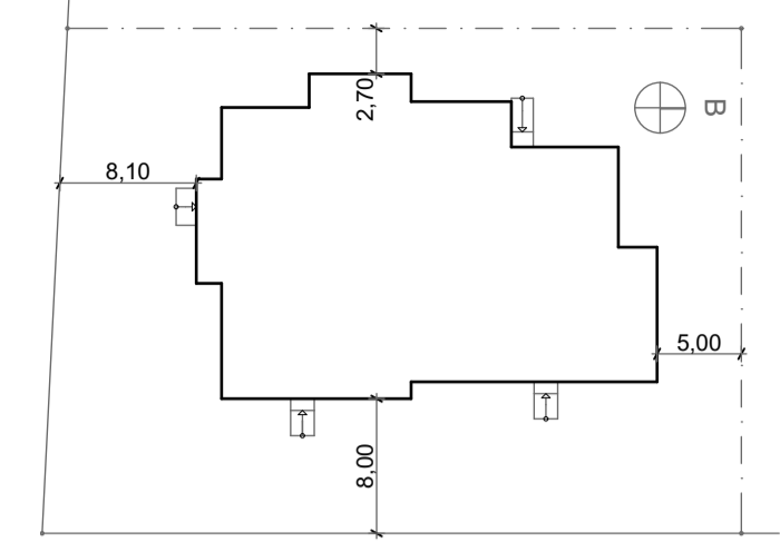
ΦΕ-01 Κλειδιά 1:500
