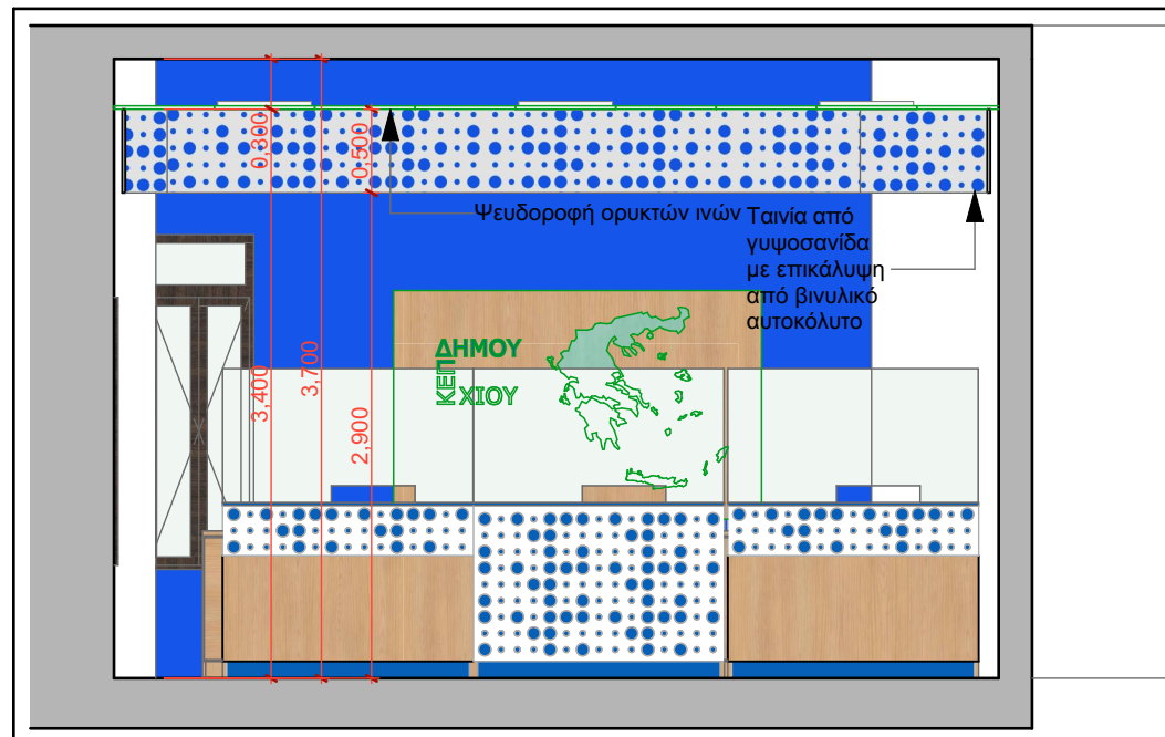
ΚΕΠ 1β Α ΚΕΠ 1 Δ.Ε. Χίου (τμήμα β) Τομή Α-Α 1:50
