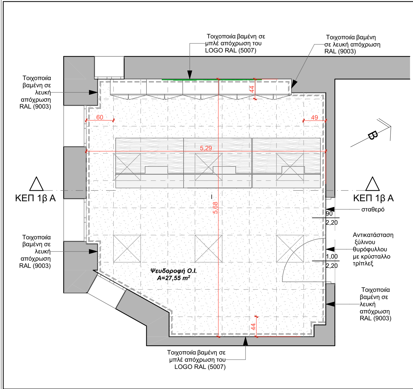
0. ΚΕΠ 1 (τμήμα β) Δ.Ε. Χίου Κάτοψη 1:50
