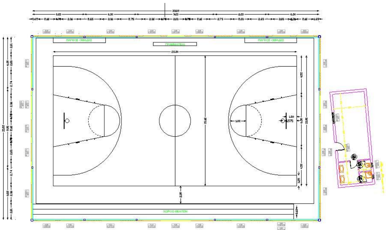
Εικόνα 1: Κάτοψη ισογείου Βούρειου Αθλητικού Κέντρου Λιβαδίων
